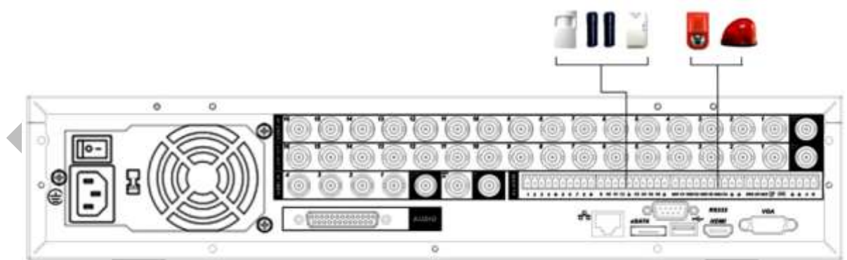
Rys. 3-5 Sposób podłączenia wejść i wyjść alarmowych.
