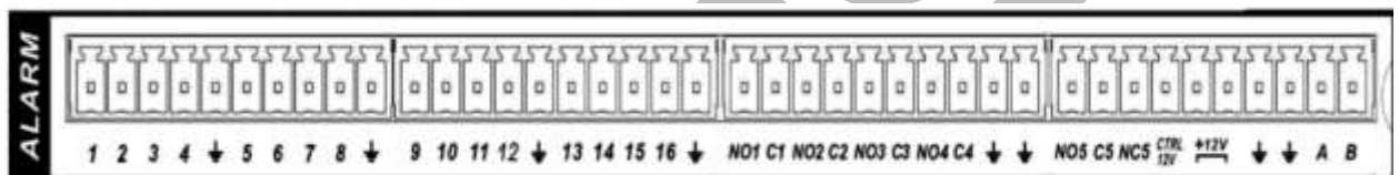
Rys. 3-6. Rozmieszczenia wejść / wyjść alarmowych rejestratora serii HE-T.
