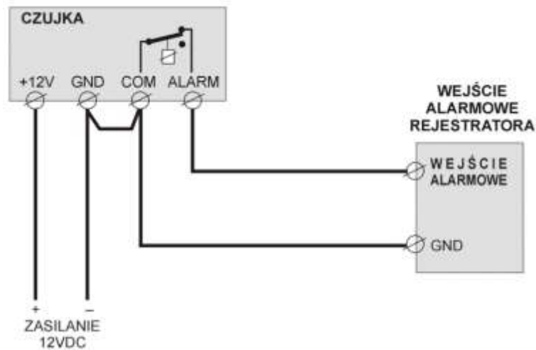
Rys. 3-7. Schemat podłączenia czujki do wejść alarmowych rejestratora.
