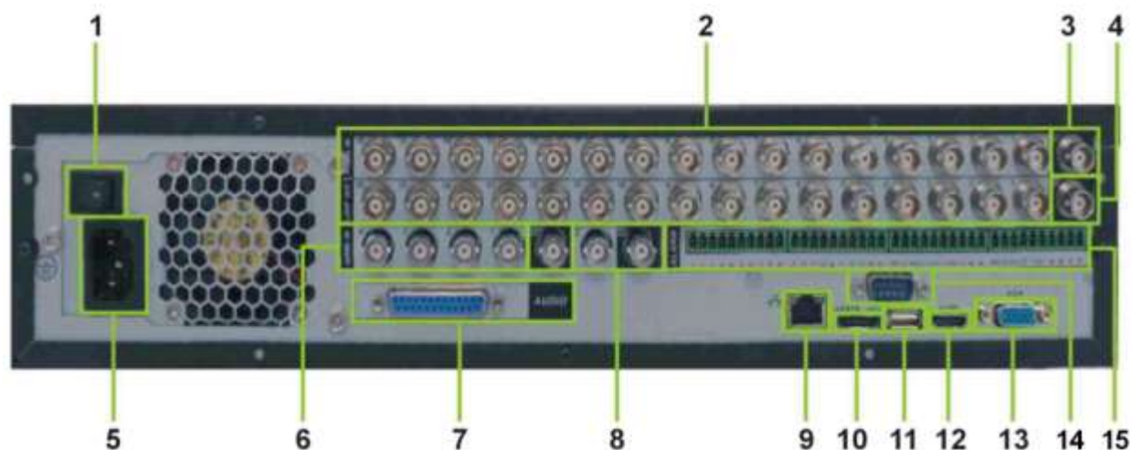
Rysunek 2-2. Wygląd panela tylnego rejestratora serii HE-T.
